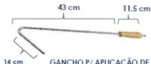
GANCHO P/ APLICAÇÃO DE VERMÍFUGO ORAL Acompanha mangueira
